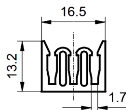
SZ-3RD/N MATERIAŁ: PVC KOLOR: szary
