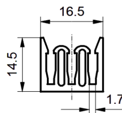
SZ-3F MATERIAŁ: PVC KOLOR: szary
