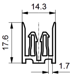
SZ-3R MATERIAŁ: PVC KOLOR: szary
