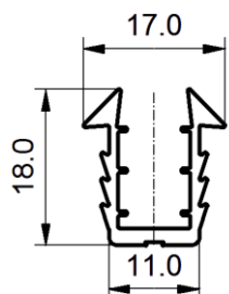
U01 MATERIAŁ: PVC MIĘKKIE KOLOR:czarny, szary
