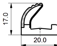
HZD20 MATERIAŁ: PVC+PVC MIĘKKIE KOLOR: czarny
