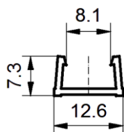
EMC MATERIAŁ: PVC KOLOR:szary
