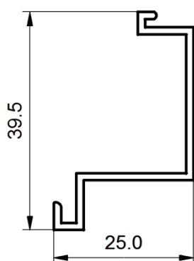
WIM03 MATERIAŁ: PVC KOLOR:czarny
