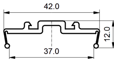
PP1 MATERIAŁ: PVC KOLOR:czarny
