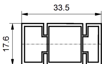
WIM01 MATERIAŁ: PVC KOLOR:czarny
